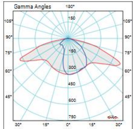
Işık Şiddeti Dağılım Eğrisi Light Distribution Curve
